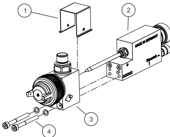
Rys. 16: Uszczelnienia iglicy
