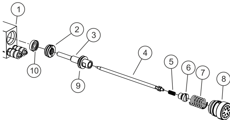
Rys. 10: Montaż iglicy materiału
